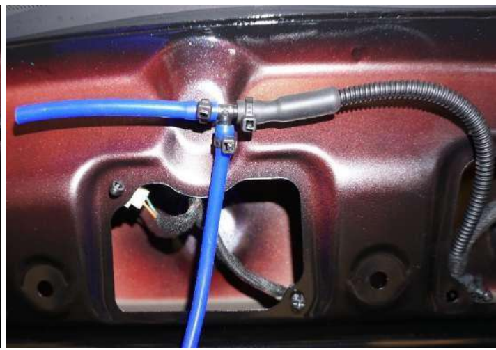
Рисунок 16 - Установка фитинга
