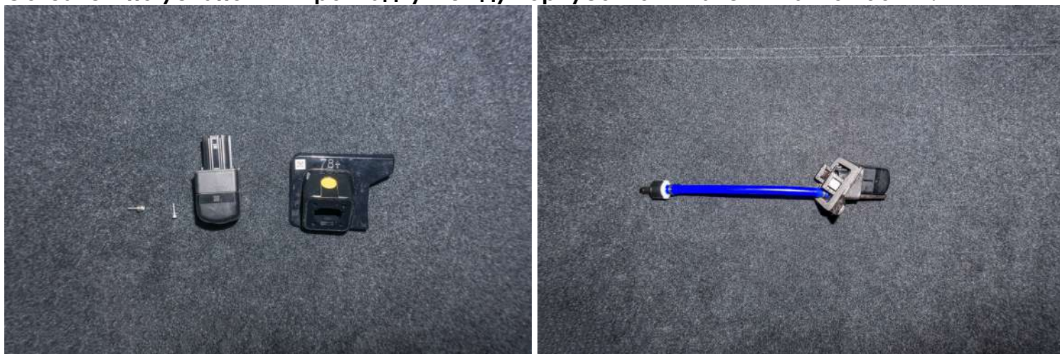
Рисунок 8 – Установка камеры заднего вида в корпус омывателя
