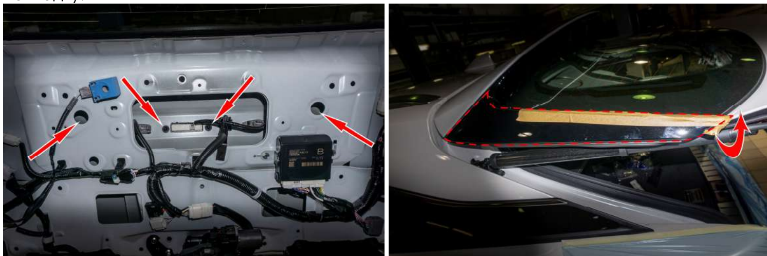
Рисунок 5 – Расположение гаек крепления внешней накладки
