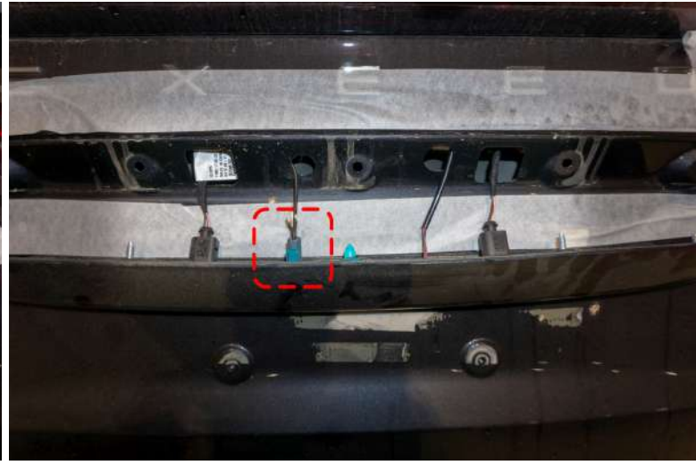
Рисунок 6 – Расположение провода питания
