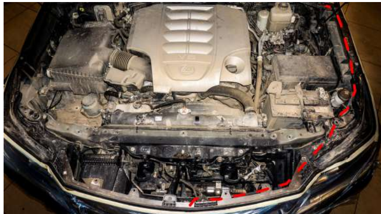
Рисунок 6 – Установка корпуса омывателя и расположение трубки
