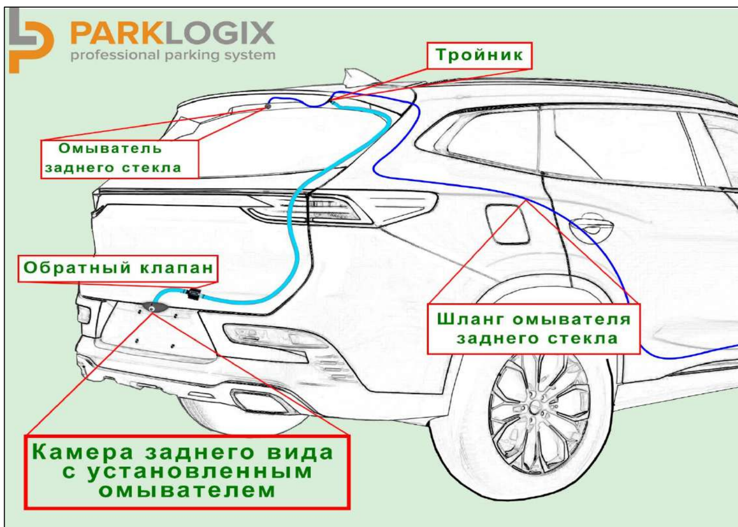
Рисунок 1. Подключение к омывателю заднего стекла.
