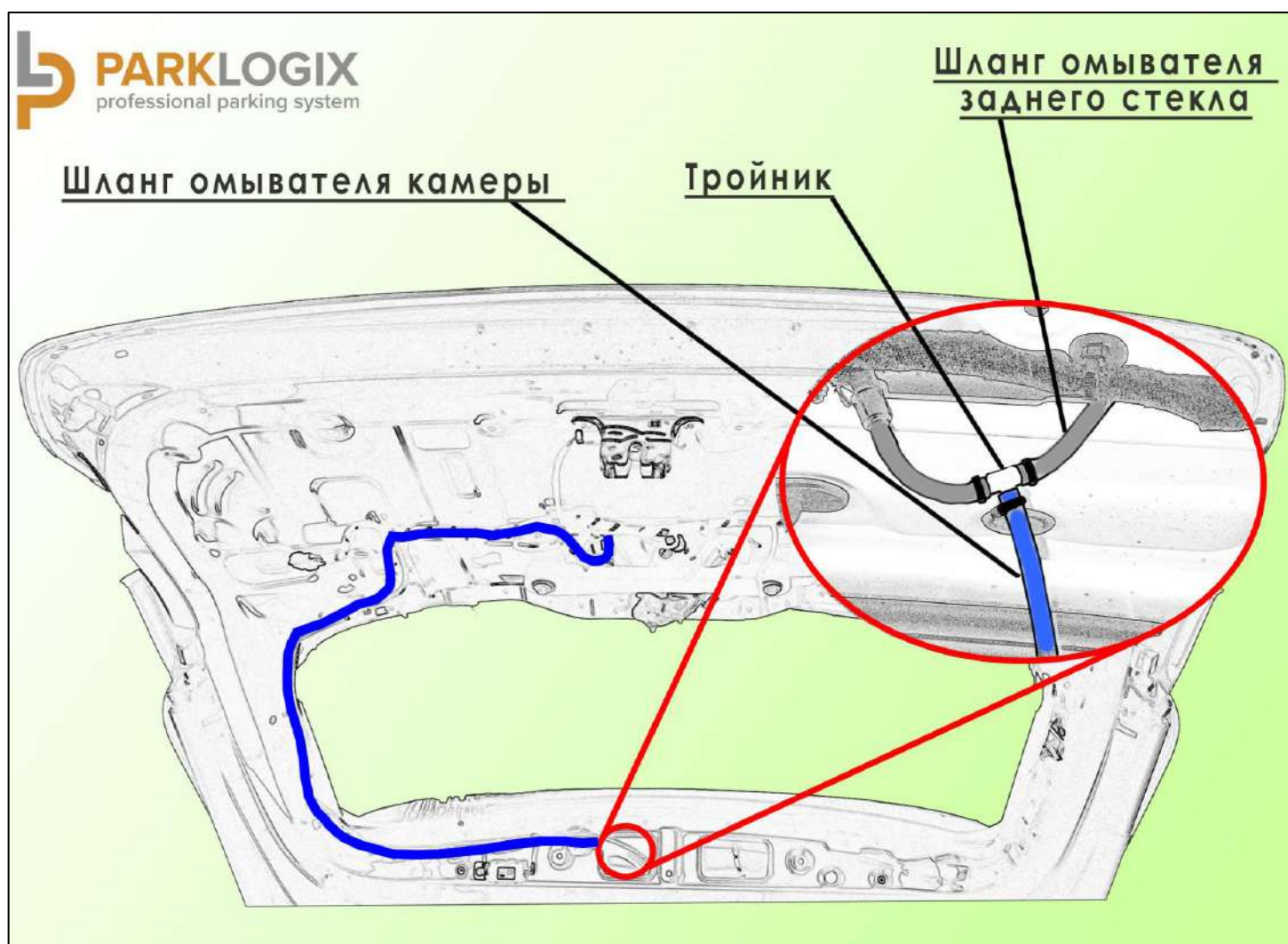
Рисунок 5. Установка тройника.
