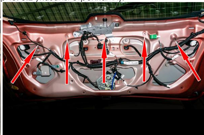
Рисунок 5 – Расположение клипс крепления
