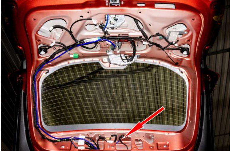
Рисунок 8 – Расположение трубки в багажном отделении
