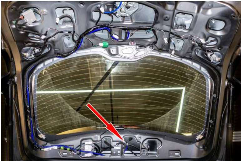
Рисунок 7 – Расположение трубки в багажном отделении
