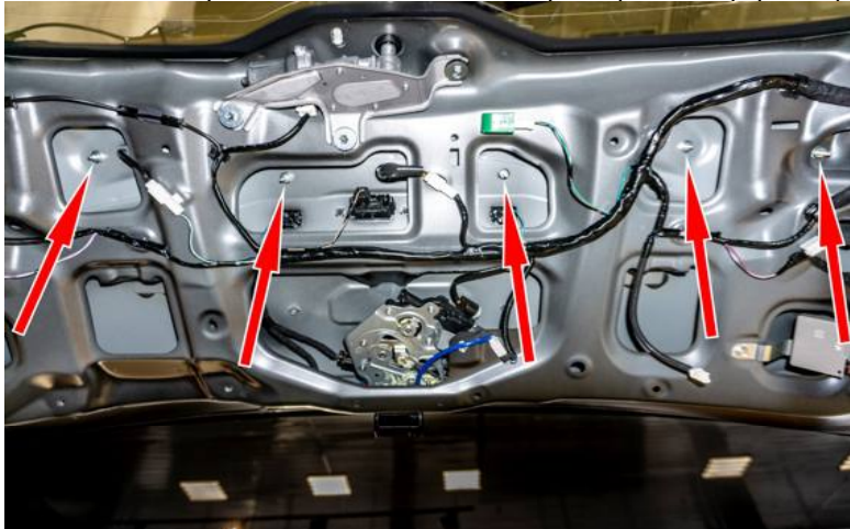
Рисунок 5 – Расположение гаек и клипс крепления
