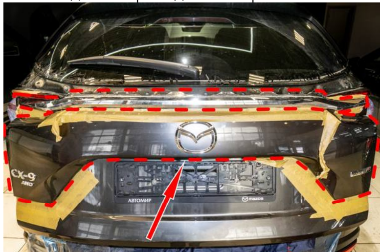
Рисунок 6 – Расположение накладок и винтов крепления
