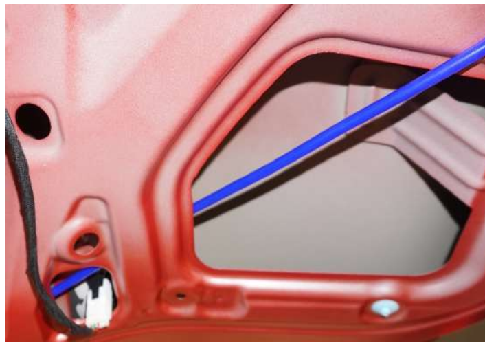
Рисунок 18 – Протяжка трубки в полости багажного отделения
