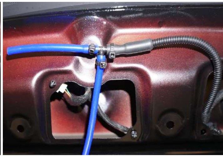
Рисунок 16 – Установка фитинга
