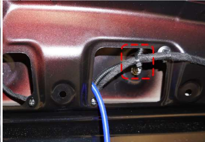
Рисунок 17 – Фиксация трубки
