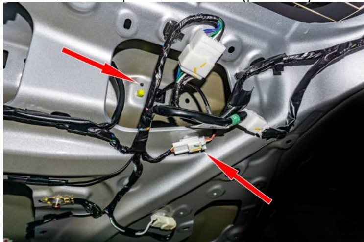
Рисунок 6 – Расположение винтов крепления и разъема
