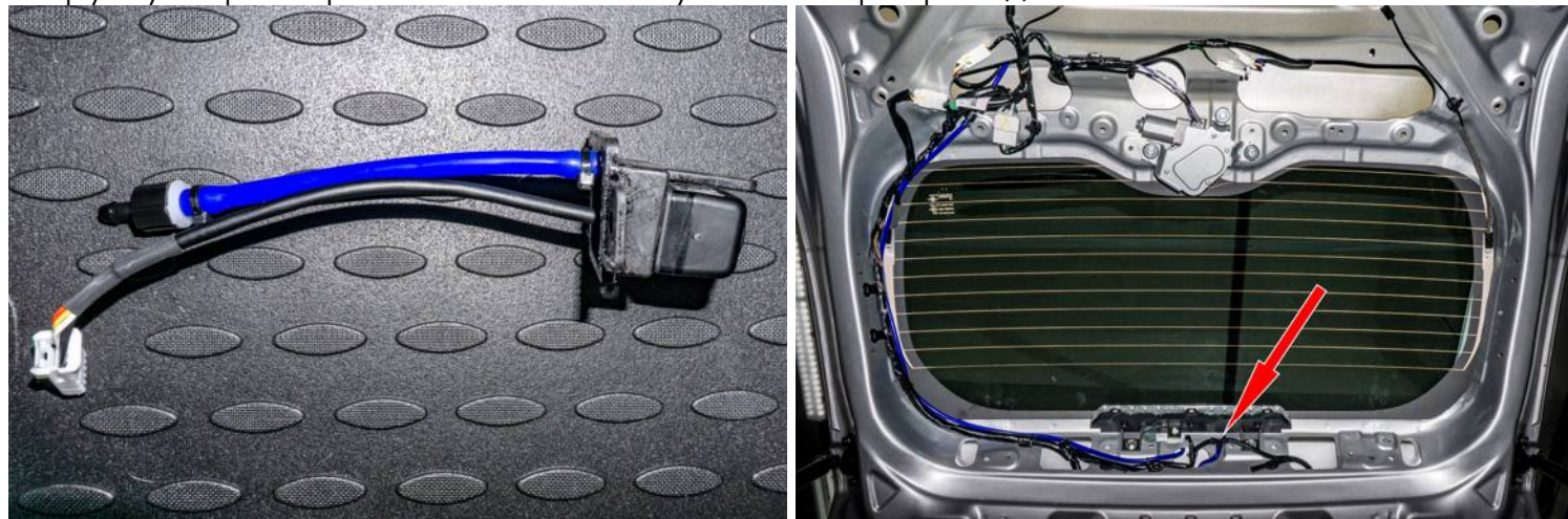
Рисунок 8 – Расположение трубки в багажном отделении
